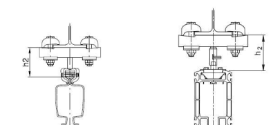
(スチールレール用) (アルミレール用)
