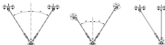
【Vサスペンション一例】
