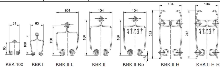
【スチールレール外形図】
